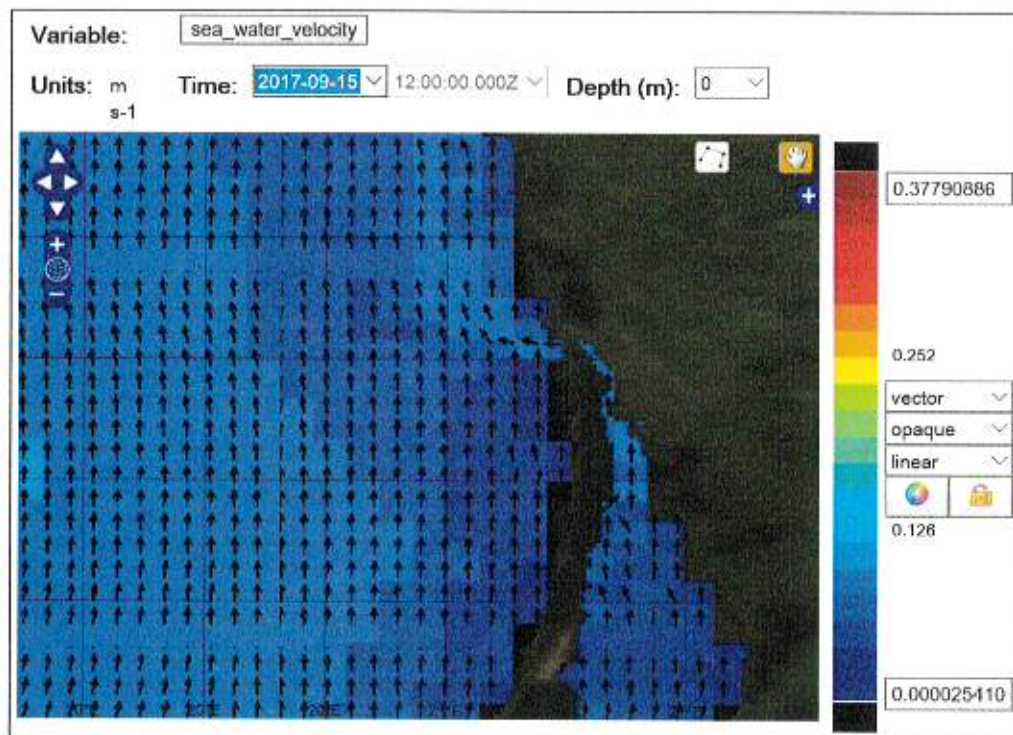
3.6.55 pav. Jūros vandens greitis dažniausiai buvo į šiaurę 2017 m. ir 2018 m. vasaromis, atitinkamai vidutinis greitis 0,13 ir 0,19 m/s. (Copernicus, 2019a).
